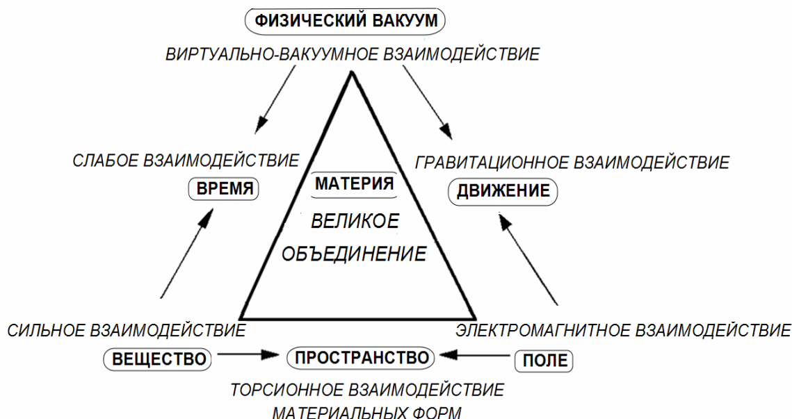
Рис. 14. Модель фундаментальных видов физического взаимодействия
