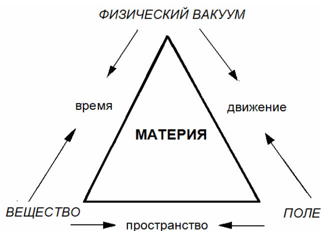
Рис. 12. Модель физической реальности
