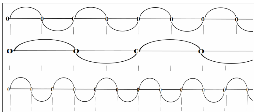
Рис. 15. Демонстрация совпадения нулей функции
