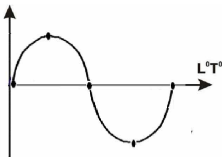
Рис. 4. Синусоидальная модель реальности в общем виде
