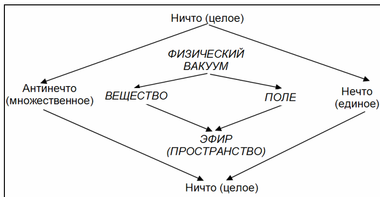
Рис. 2. Модель генезиса реальности
