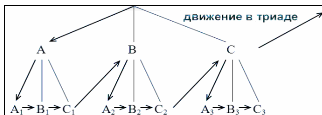
Рис. 6. Гегелевская триада: реализация триадного принципа развития
