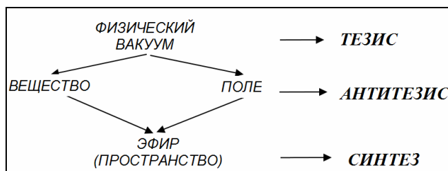
Рис. 3. Триадная модель генезиса реальности
