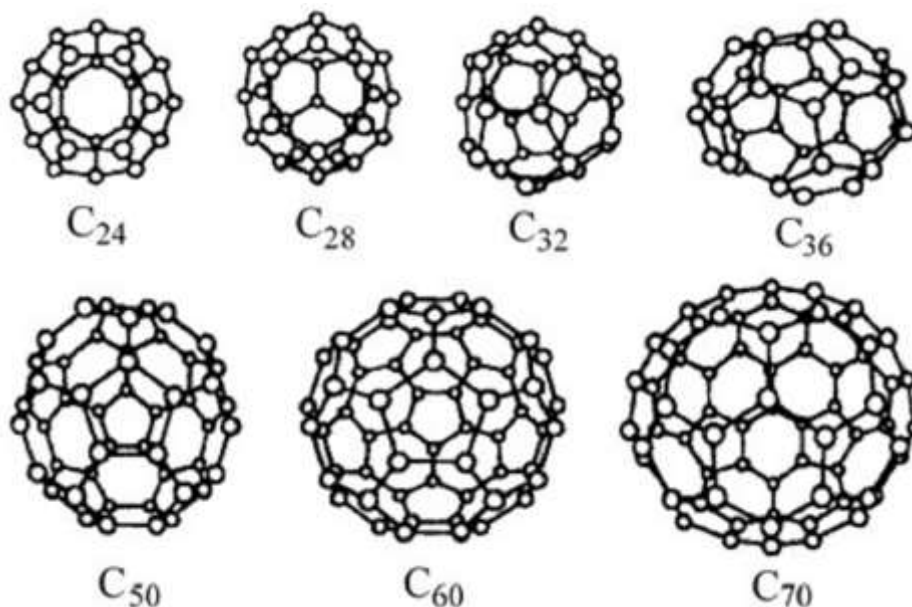
Рис. Небольшие по размерам фуллерены обладают уникальной особенностью – они повторяют сферическую форму исходного элемента – сферического атома углерода. Наибольший из сферических – фуллерен C_{60}
