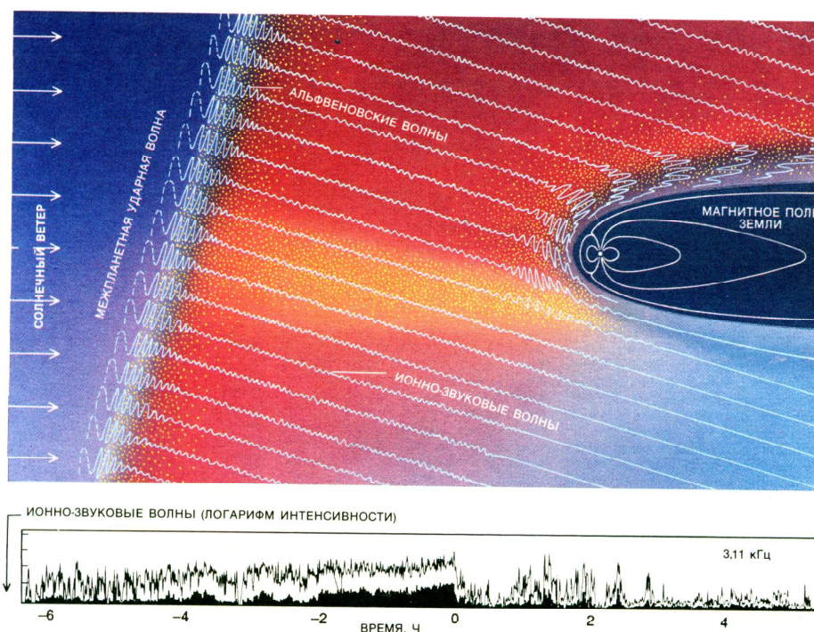
Рис. 1. Формирование ударной волны, магнитной волны и ионно-звуковой волны при встрече гиперзвукового потока солнечной плазмы с магнитосферой Земли. (Scientific American. №6. 1991).
