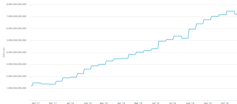
Изменение сложности майнинга биткоина
