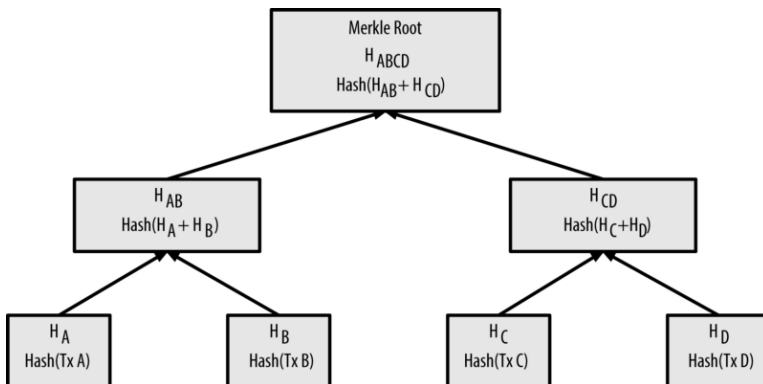
Дерево Мёркла
