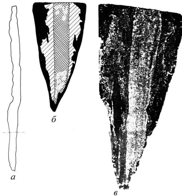
Рис. 3. Трёхслойный нож из Бирки (по В. Arrhenius and L. Tapper): а – нож; б – технологическая схема; в – фотография микроструктуры.
