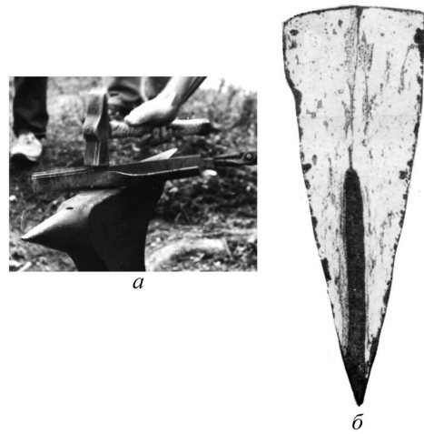
Рис. 2. Способ формовки трёхслойной заготовки (второй вариант):
