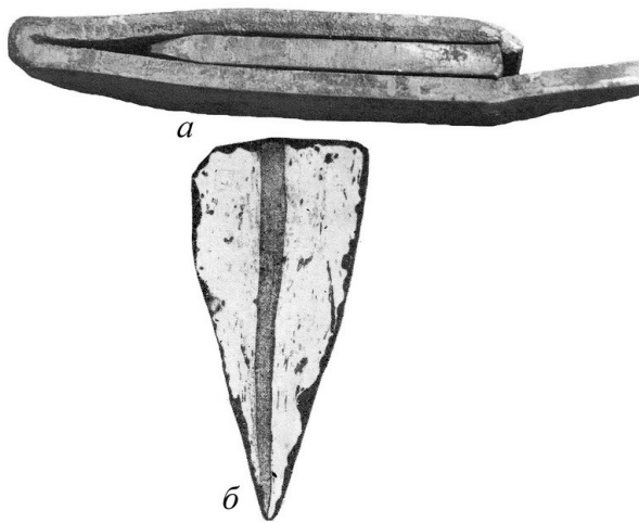
Рис. 1. Способ формовки трёхслойной заготовки (первый вариант):
